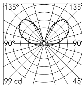
Luminous flux luminaire 898 lm
