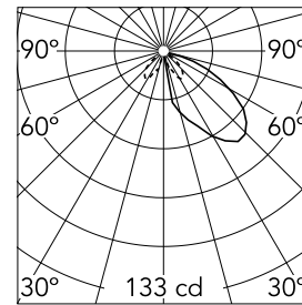
Luminous flux luminaire 317 lm
