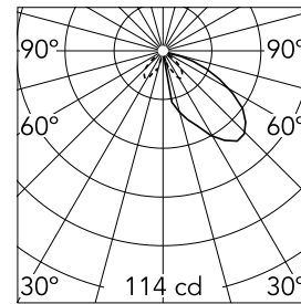
Luminous flux luminaire 272 lm
