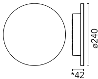
*Concrete, crema d'orcia, basaltina H = 48 mm
