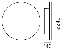
*Concrete, crema d'orcìa, basaltina H = 48 mm
