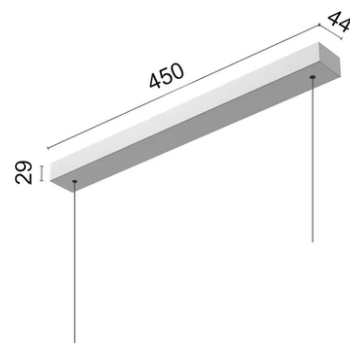
Surface Kit 60W. Non Dimmable 08.0520.02
